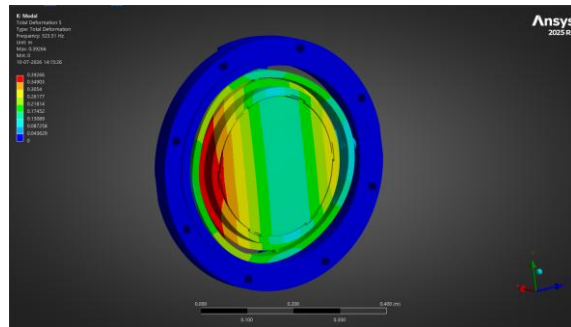
Mode 5 — 523.51 Hz
