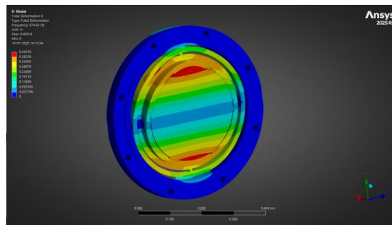
Mode 6 — 674.63 Hz
